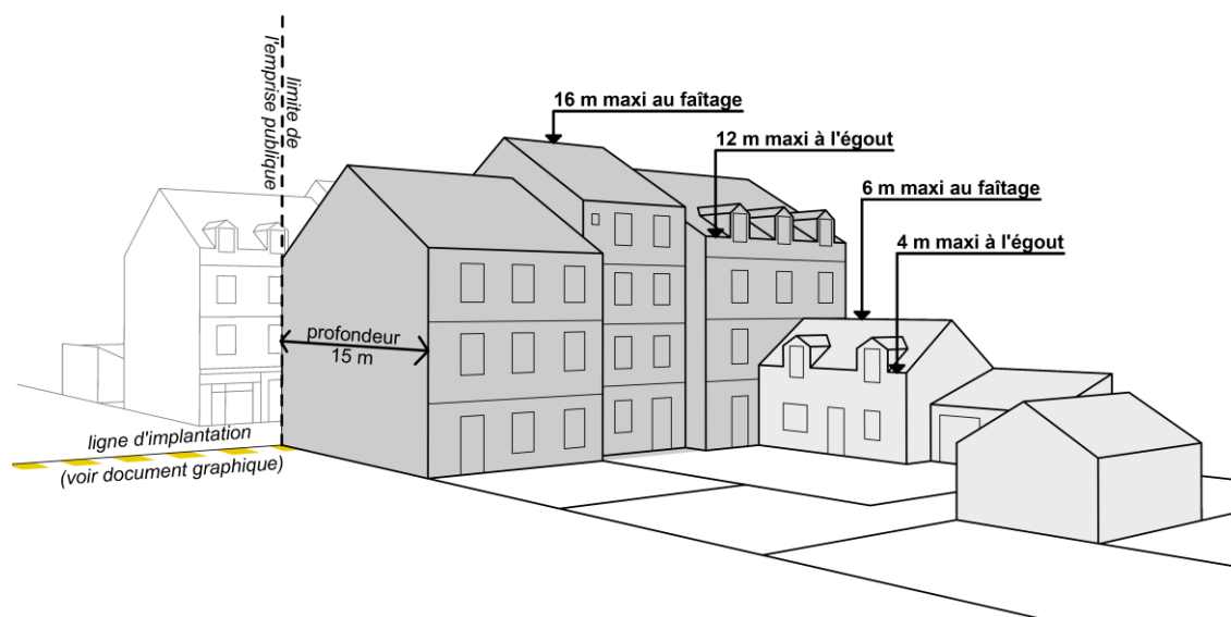
Hauteur des constructions dans le cas des implantations bâties de type 1
