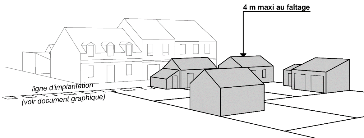
Hauteur des constructions dans le cas des implantations bâties de type 3
