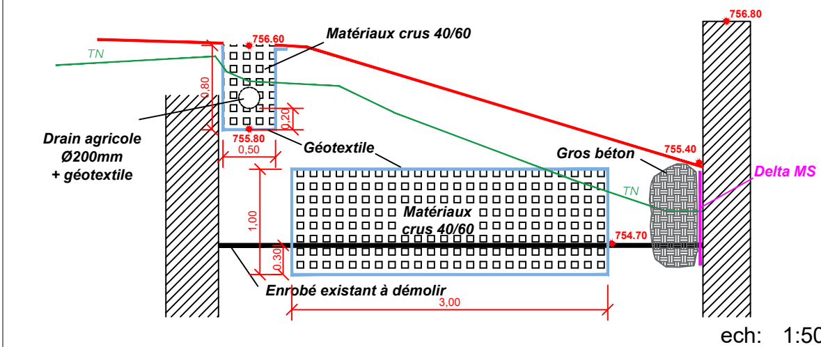
Ouvrage d'infiltration - COUPE BB - Matériaux crus sur 3x3x1m sous espaces verts
