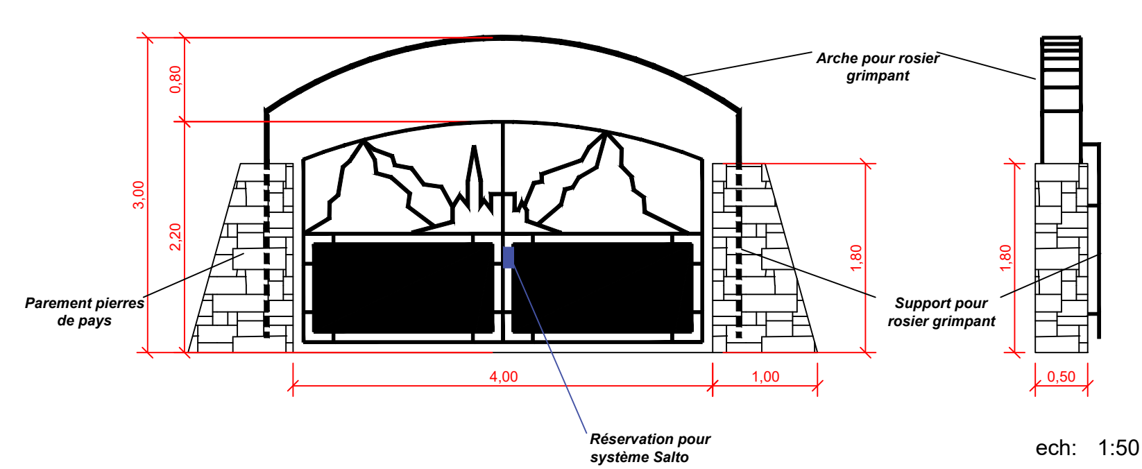
Détail portail entrée
