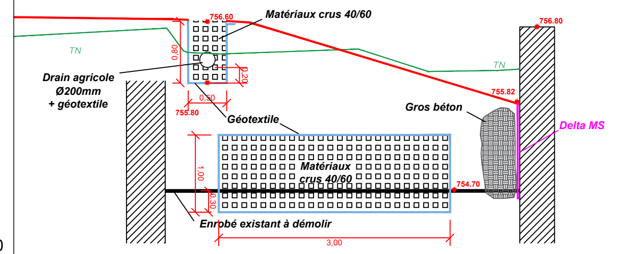
Ouvrage d'infiltration - COUPE CC - Matériaux crus sur 3x3x1m sous espaces verts
