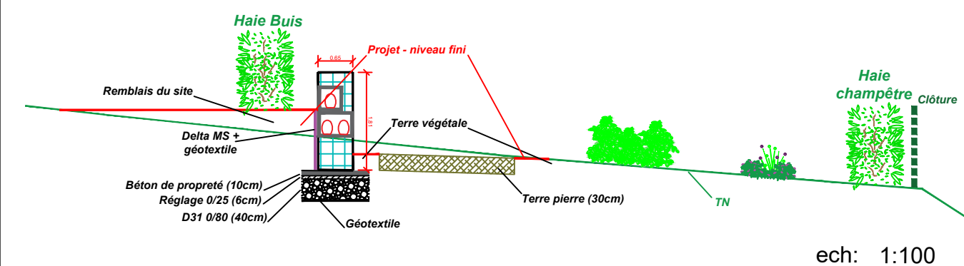
COUPE AA - GABION / COLUMBARIUM
